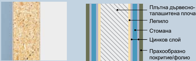
Плътна дървесно-талашитна плоча по желание
