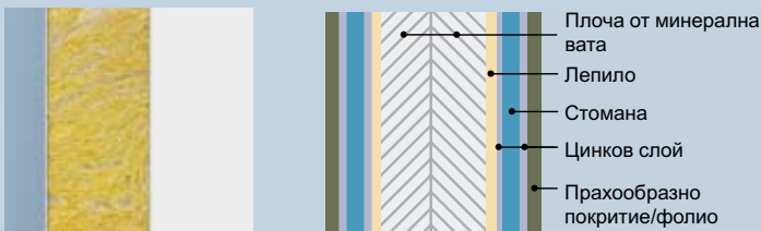
Плоча от минерална вата по желание
