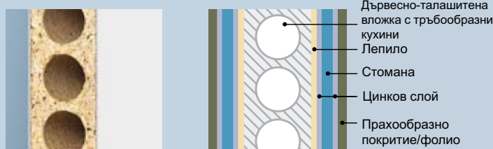
Серийна дървесно-талашитна плоча с отвори
