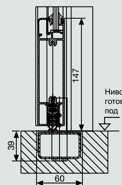
Без долен фалц (за серията, по желание с автоматично спускащо се към пода уплътнение).
