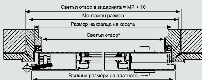
С ъглова каса
