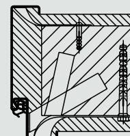
Ограждаща каса Монтаж в зидарията Анкерен дюбел
