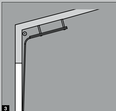
Окачване тип HD със следване на тавана
