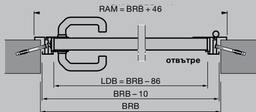
Странична врата с алуминиева ъглова каса, профил тип 3 Външен ограничител
