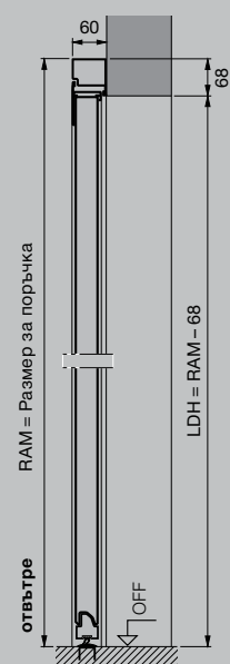
Странична врата с алуминиева блок-каса, профил тип 2 Монтаж зад отвора
