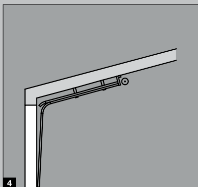
Окачване тип LD със следване на тавана
